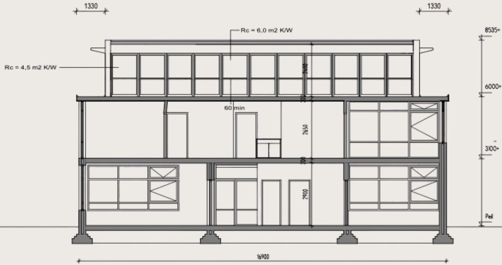
doorsnede
