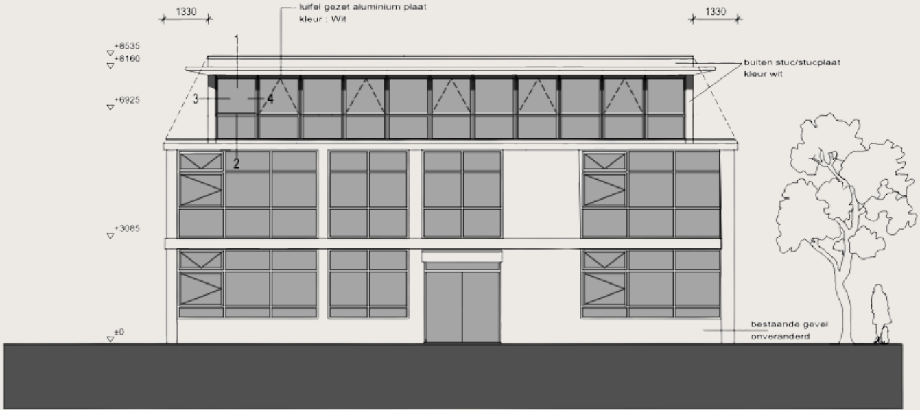
voorgevel
